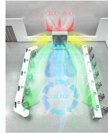
旋转射流气流图
